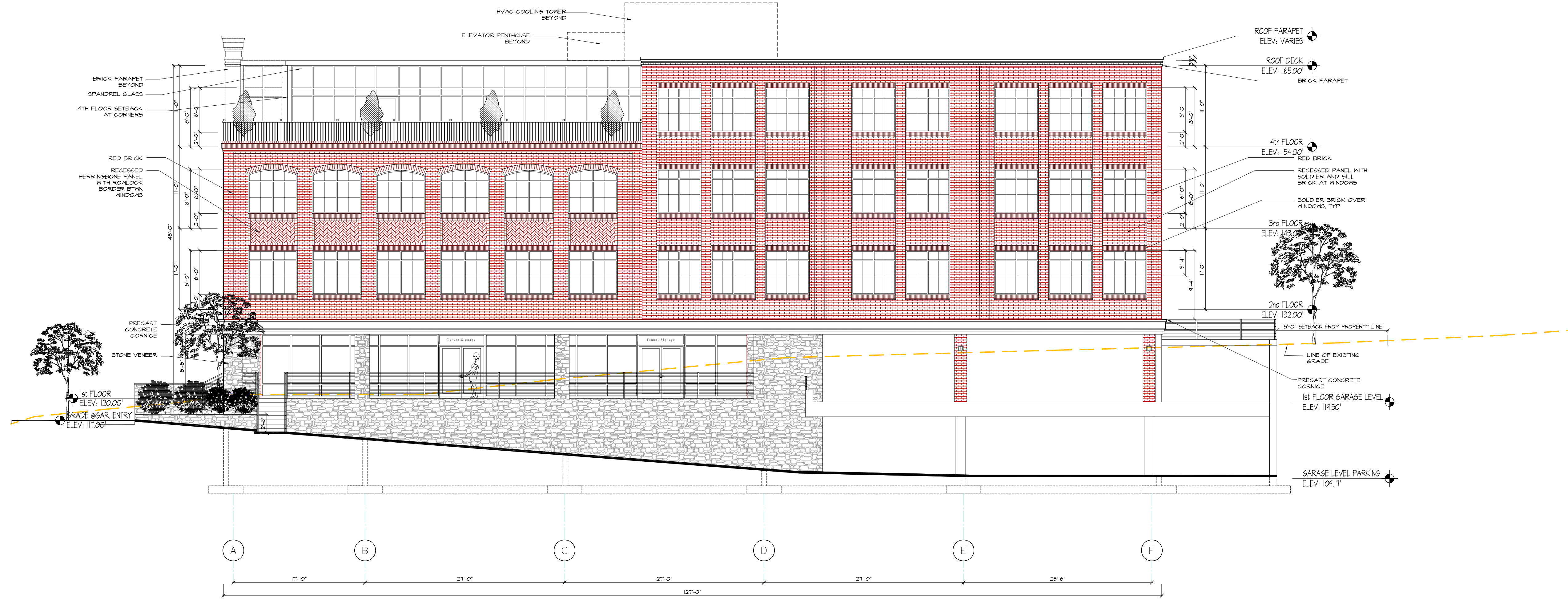
4 SOUTH ELEVATION SCALE: 1/8" = 1'-0"
